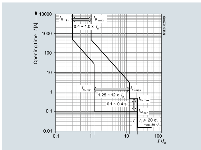
配备 ETU35WT 电子脱扣器的 3WT8 断路器，LSI 特性曲线
