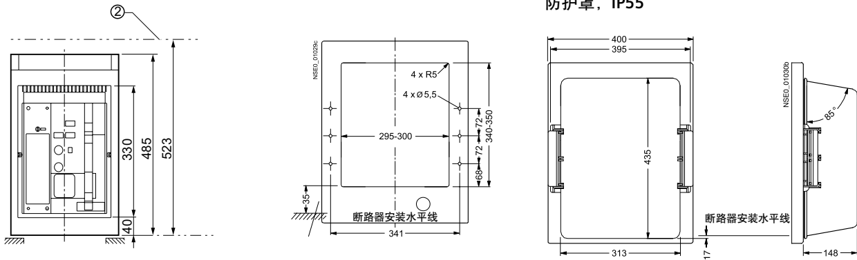
② 带灭弧罩的尺寸
