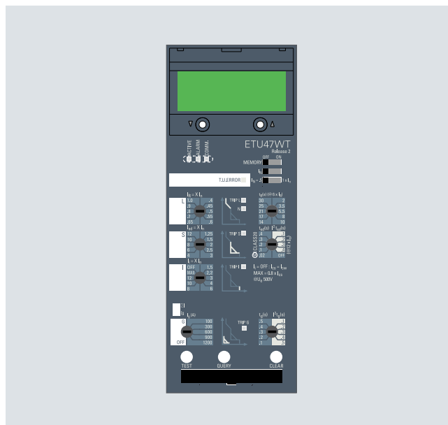
电子脱扣器
