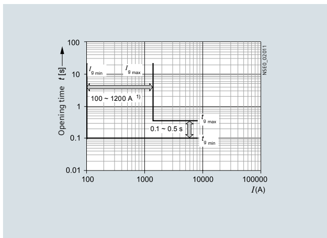
配备 ETU37WT 电子脱扣器的 3WT8 断路器，G 特性曲线 2)
