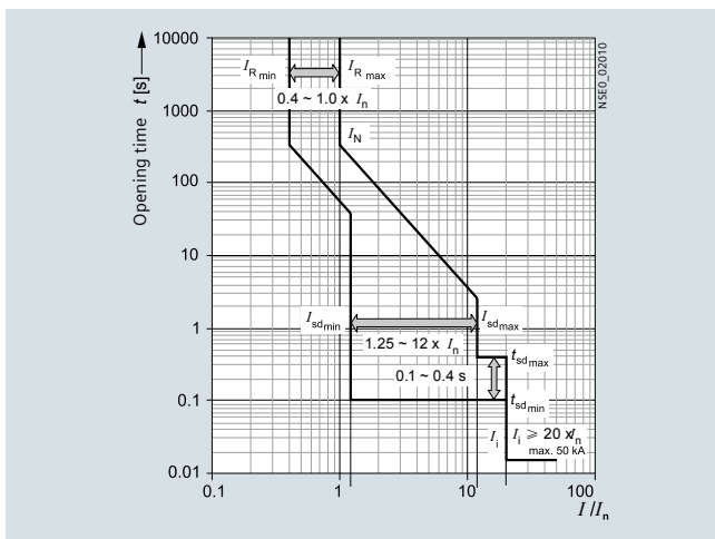
配备 ETU37WT 电子脱扣器的 3WT8 断路器，LSIN 特性曲线
