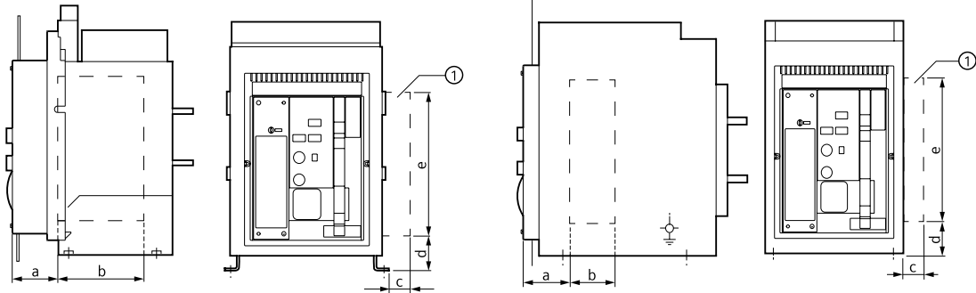
① 互锁模块的间隙 (无鲍登线)
