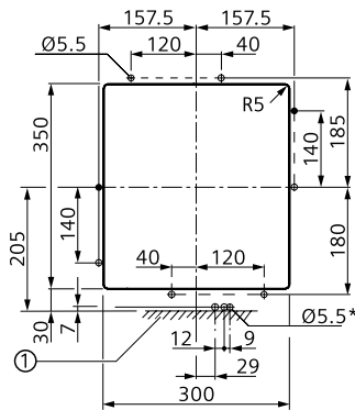
柜门开口尺寸 3 极 / 4 极 带密封框的操作员面板的门切口
