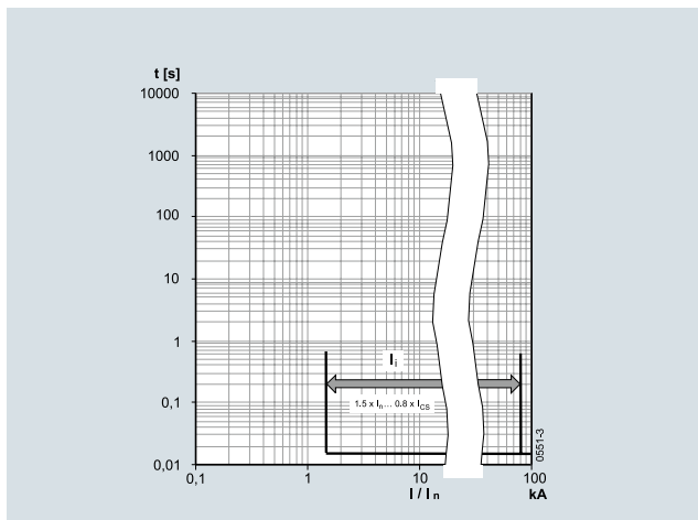
配备 ETU45WT 和 ETU47WT 电子脱扣器的 3WT8 断路器，I 特性曲线
