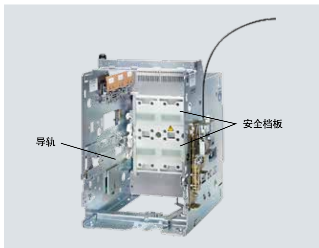
导向框架
