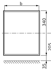
带边缘保护的门切口 在引入边缘保护后的门切口
