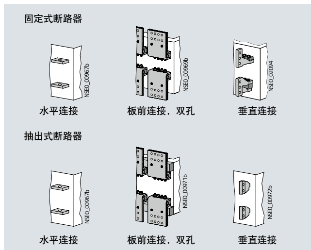
主回路连接母排
